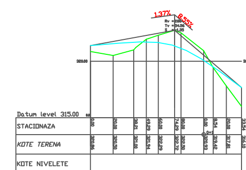
UZDUŽNI PROFIL: VC-1
