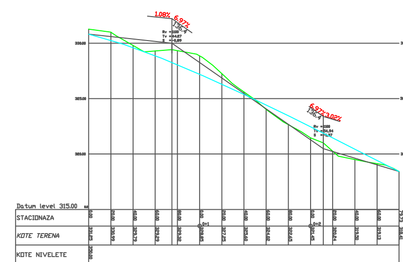
UZDUŽNI PROFIL: S-1
