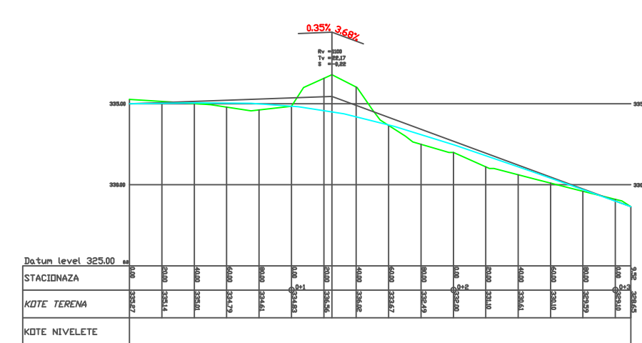
UZDUŽNI PROFIL: S-3
