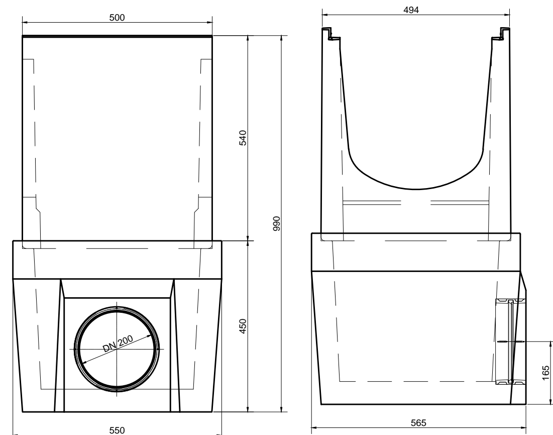
4. Taložnik: G 22194
