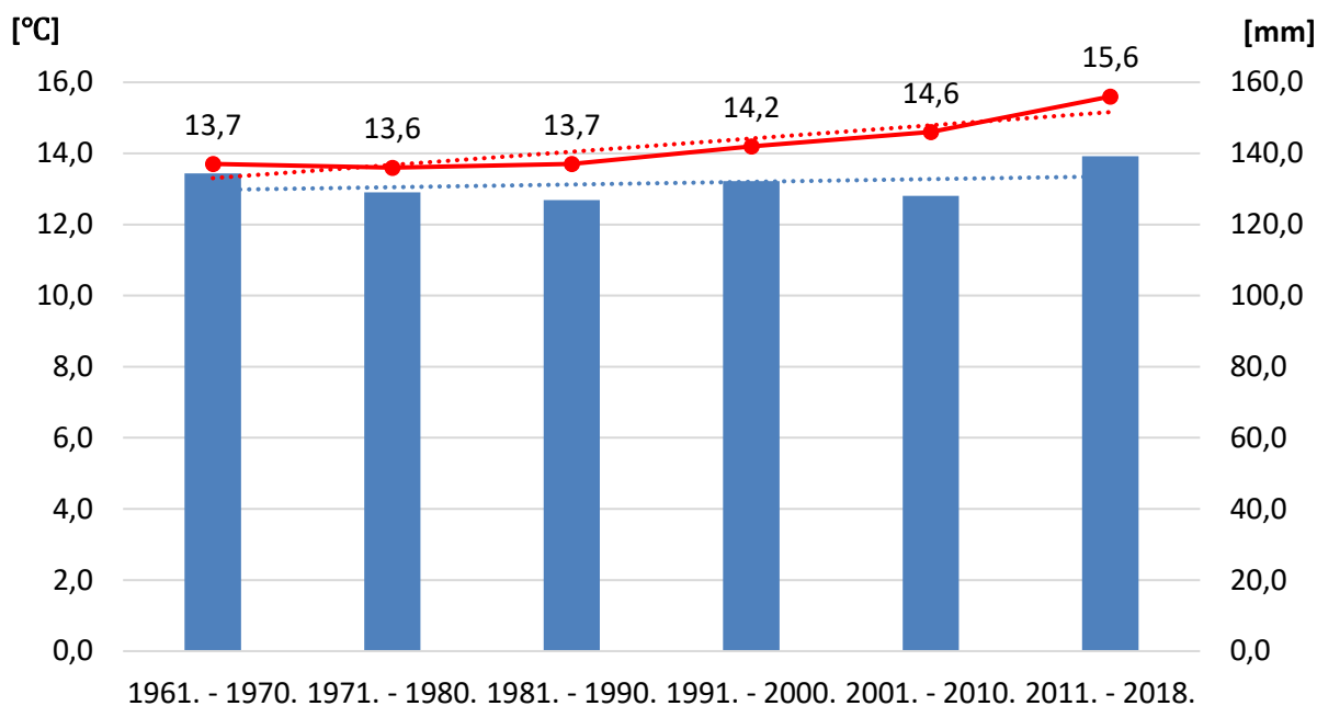
Slika 9 Srednje temperature zraka i srednje količine oborina po desetogodišnjim razdobljima od 1961. do 2018. godine
