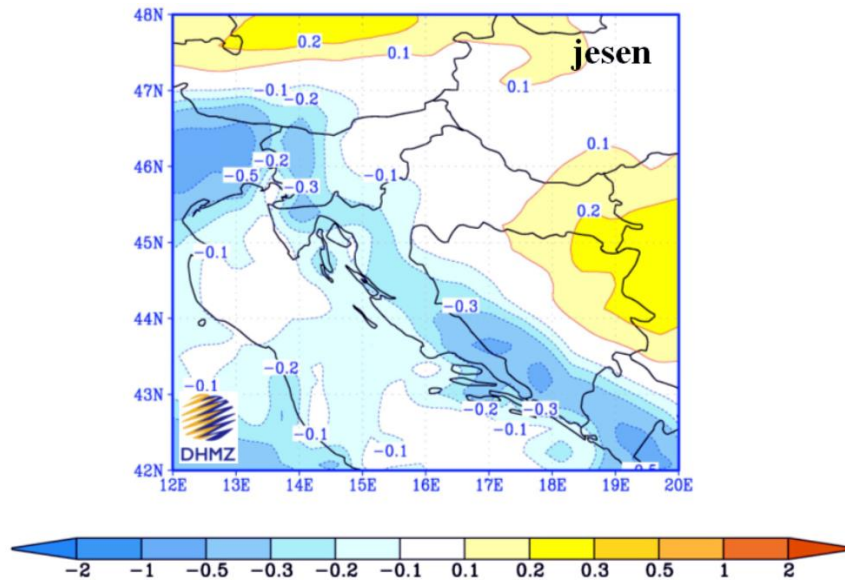
Slika 6 Promjena oborine u Hrvatskoj (u mm/dan) u razdoblju 2011. – 2040. u odnosu na razdoblje 1961. – 1990. prema rezultatima srednjaka ansambla regionalnog klimatskog modela RegCM za A2 scenarij emisije plinova staklenika za jesen.
