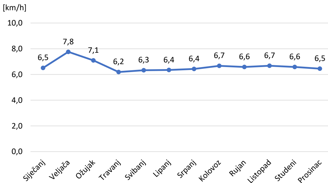
Slika 15 Srednja mjesečna brzina vjetra od 2009. do 2018. godine
